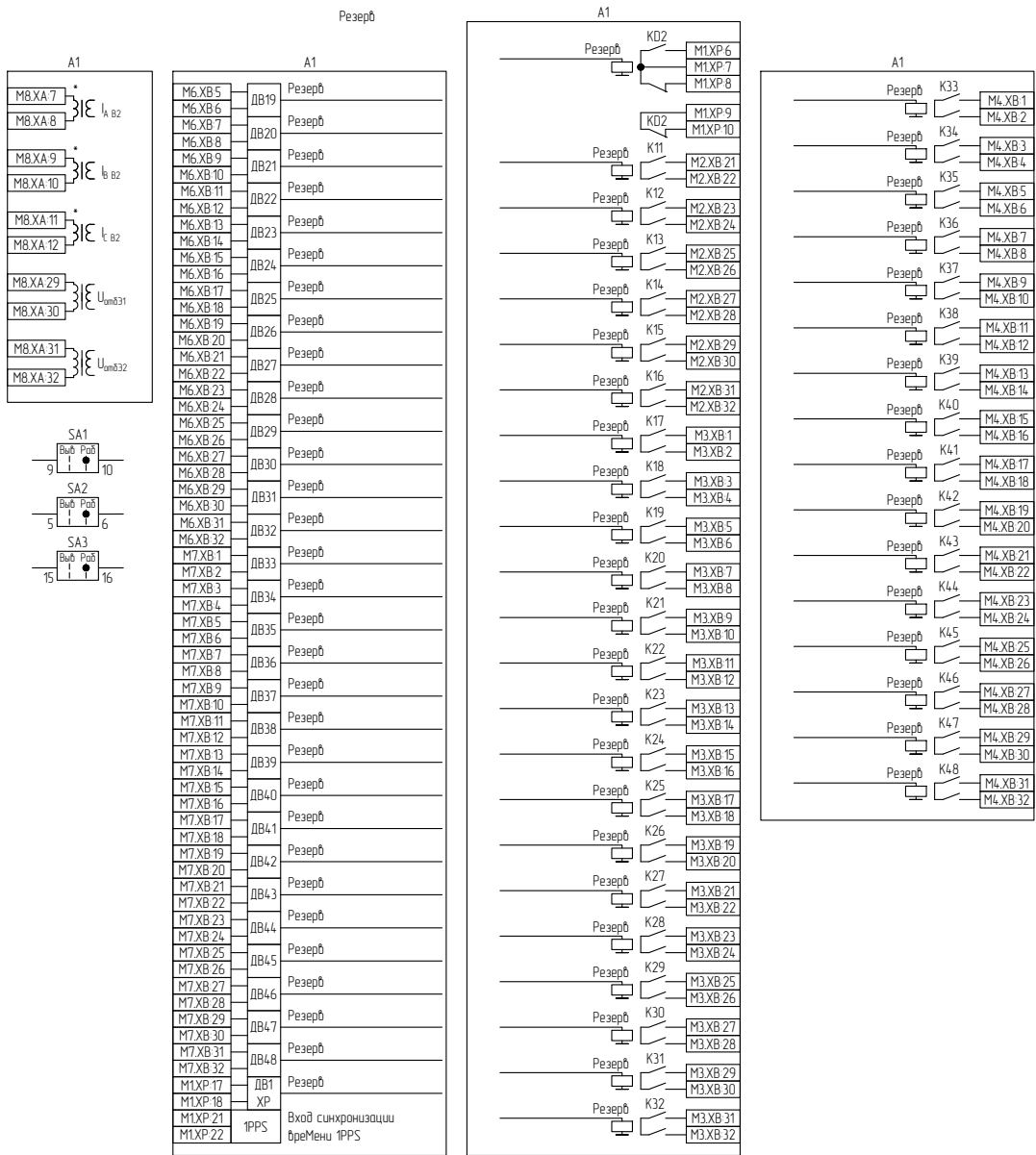
Рисунок Г.3 – Схема электрическая принципиальная (часть 3)
